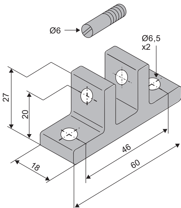
Кронштейн для крепления на створке
