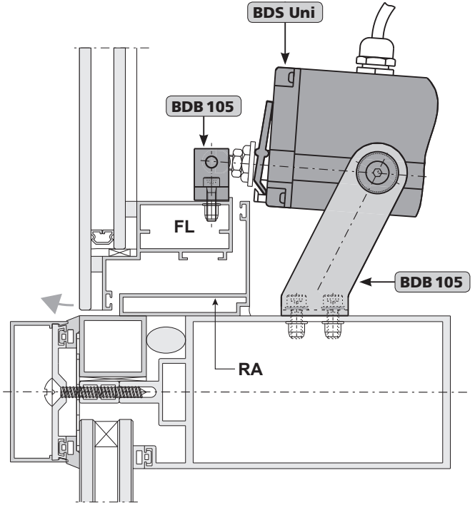
Вид установки на алюминиевом окне
