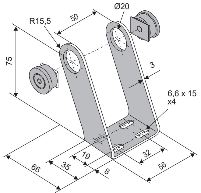
Кронштейн для крепления на раме
