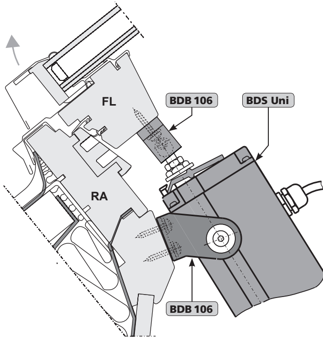
Вид установки на деревянном мансардном окне
