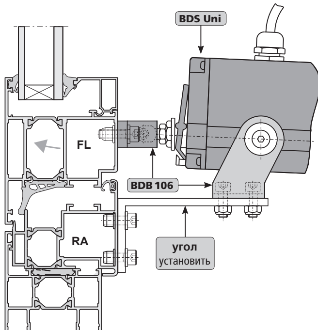
Вид установки на алюминиевом окне
