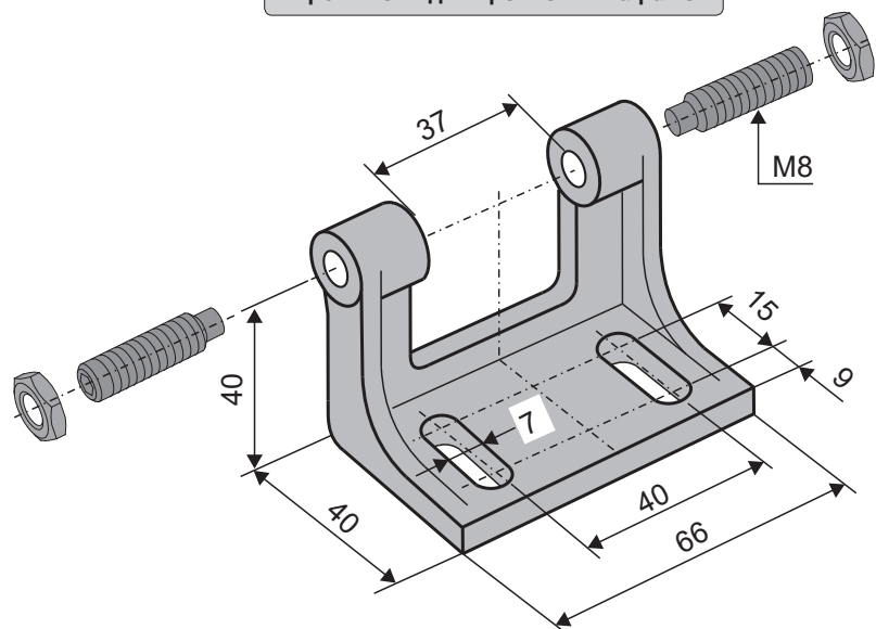
Кронштейн для крепления на раме
