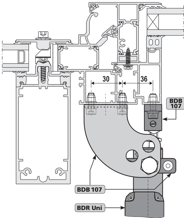
Вид установки на алюминиевом окне
