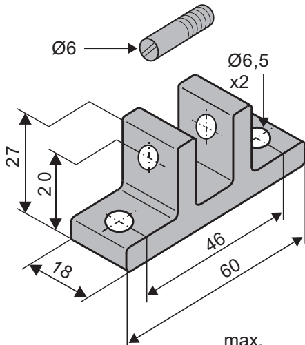
Кронштейн для крепления на створке
