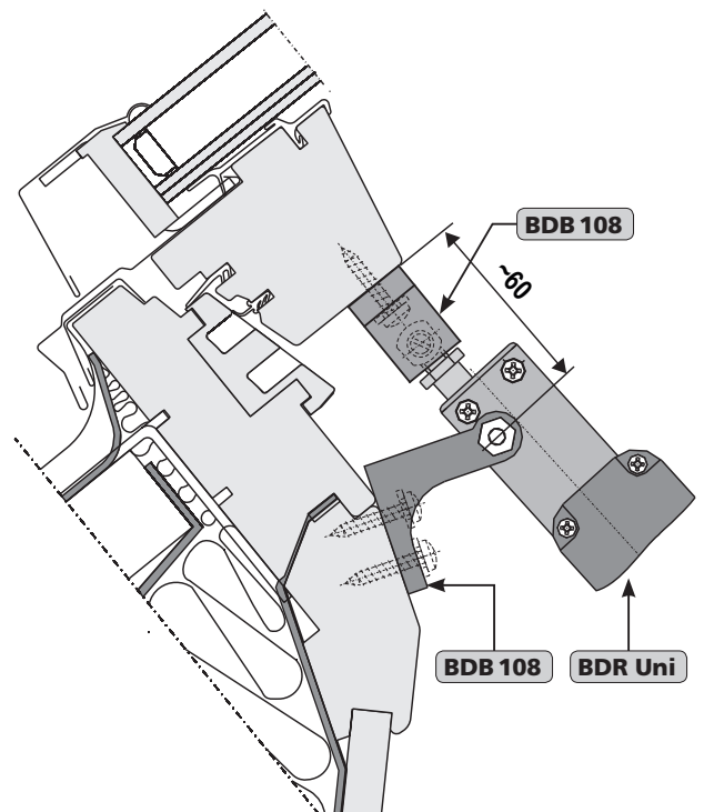
Вид установки на деревянном окне
