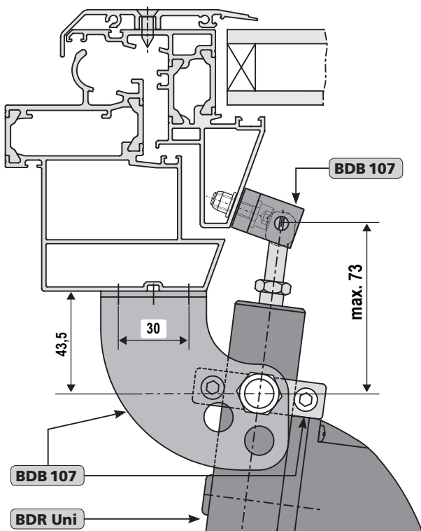
Вид установки на алюминиевом окне
